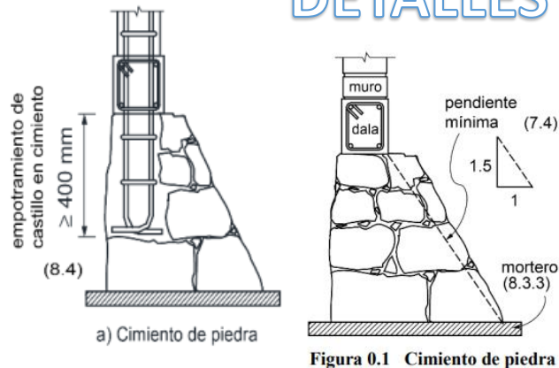
Figura 0.1 Cimiento de piedra
