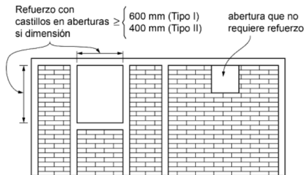
Figura 0.3 Refuerzo en el perímetro de aberturas
